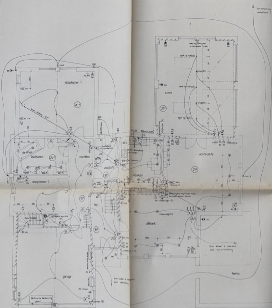
verdiepingsplan
